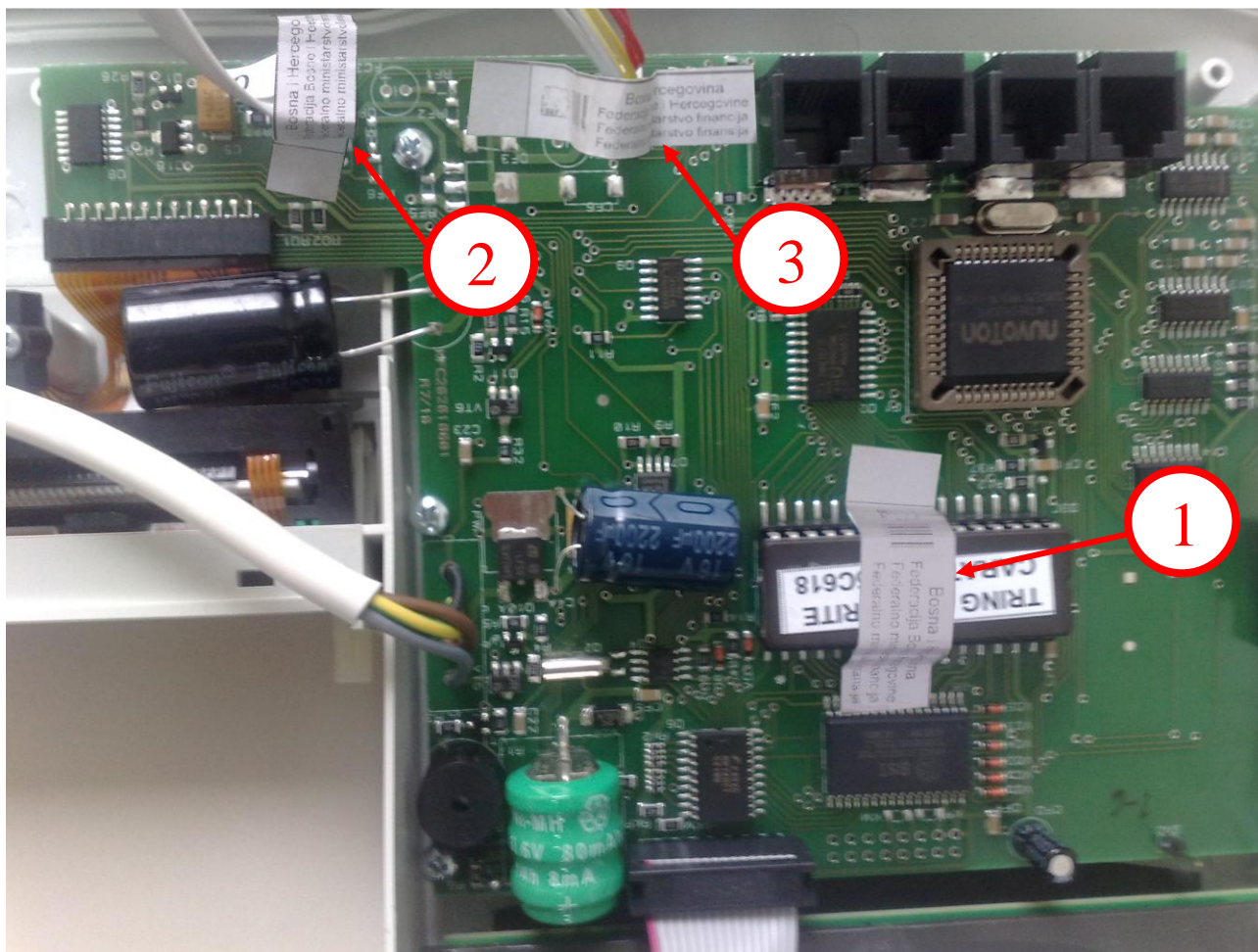
Slika 3 – Postavljanje fiskalne i programske plombe te plombe elektronskog žurnala
