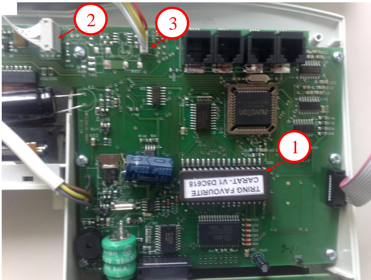
Slika 2- Mjesta za postavljanje fiskalne i programske plombe
